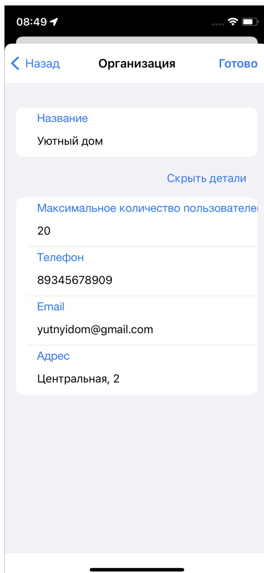
Рис. 2.57: Редактирования организации
