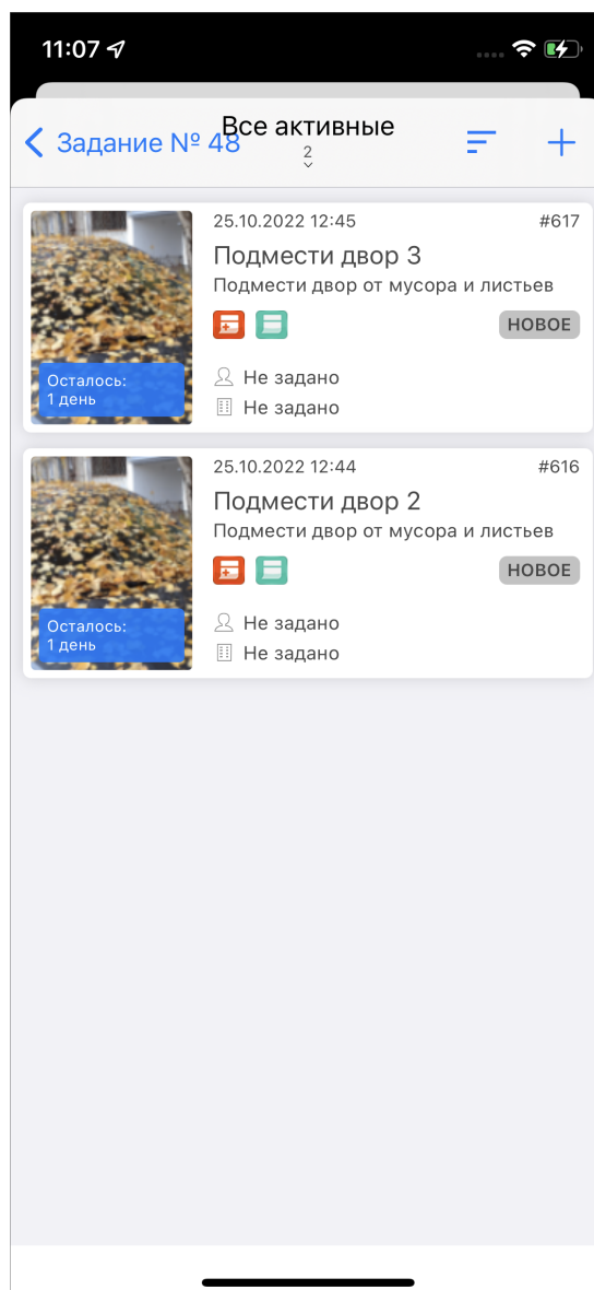
Рис. 2.45: Дочерние задания
