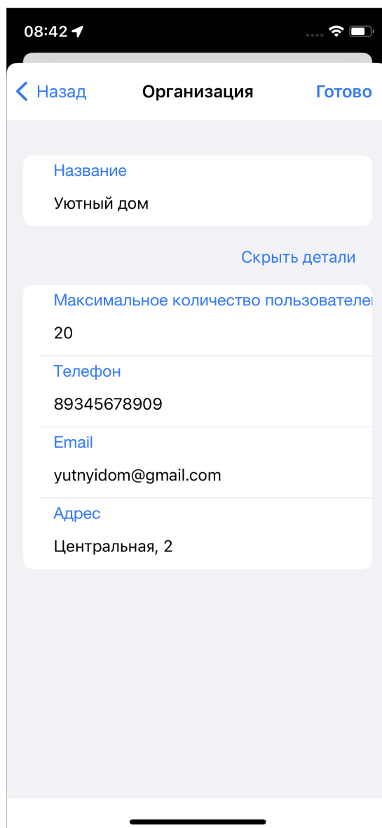
Рис. 2.55: Создание организации
