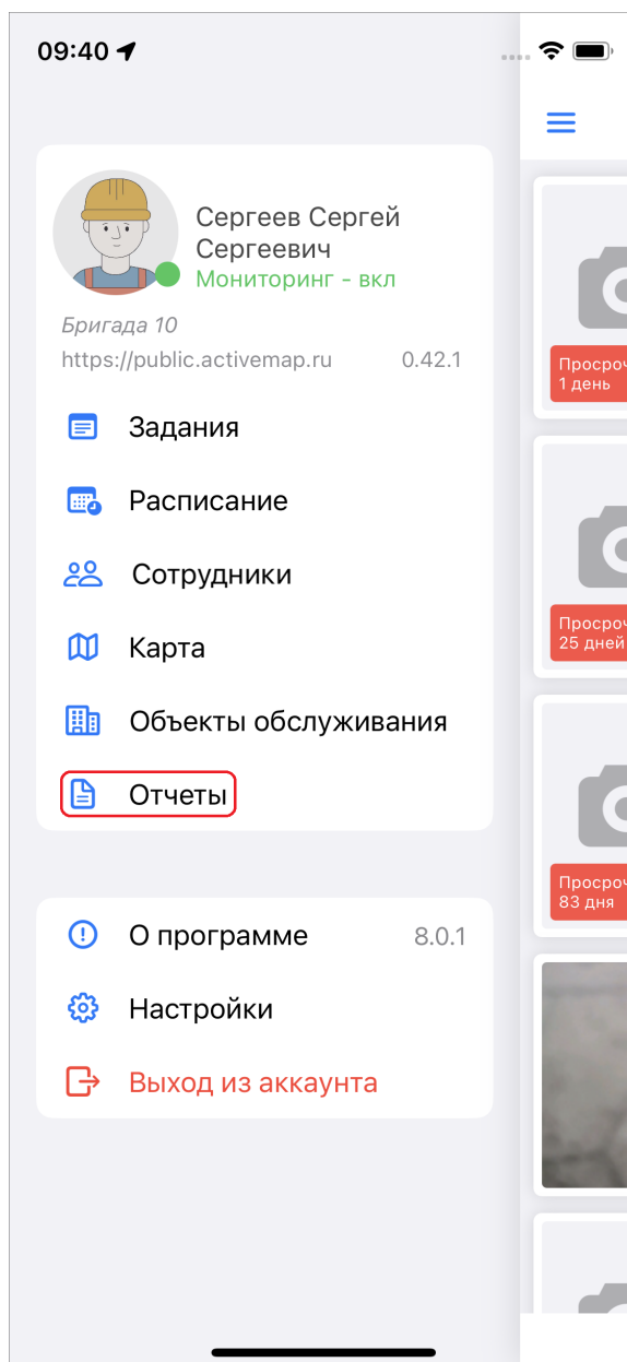
Рис. 2.95: Меню «Отчеты»
