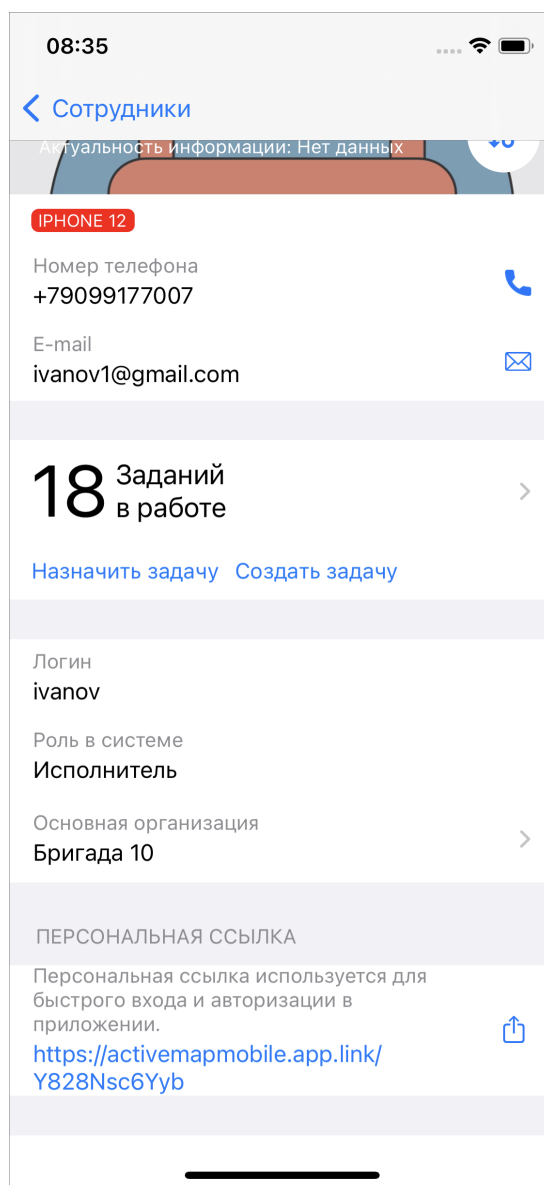
Рис. 2.47: Профиль сотрудника
