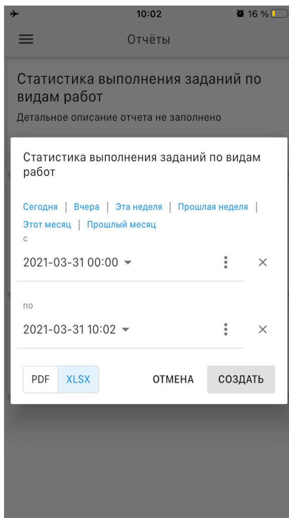
Рис. 2.97: Сформировать отчет
