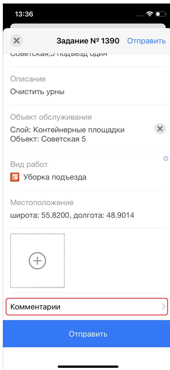
Рис. 2.42: Раздел «Комментарии»
